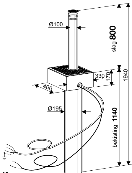
10 meter kabels Elektromotor en Eindschakelaars CORAL 1080 - gewicht 104 Kg
