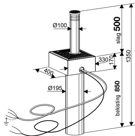
10 meter kabels Elektromotor en Eindschakelaars CORAL 1050 - gewicht 86 Kg
